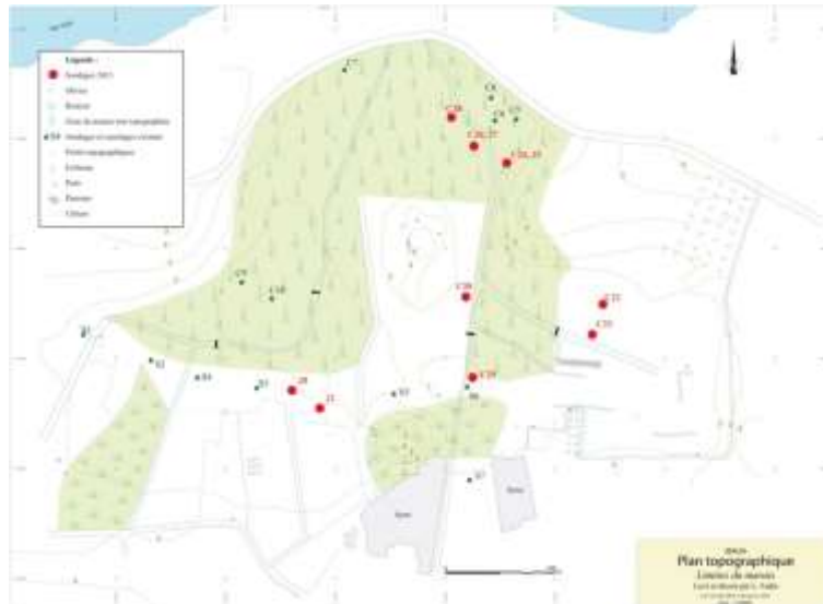
Figure 43 : Malia, étude géomorphologique du marais
